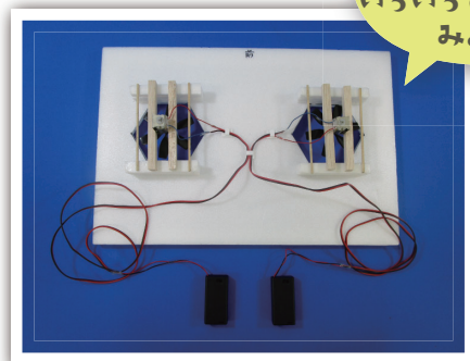
ホバークラフトの完成基本形
